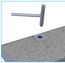
Vis de décollement pour faciliter l'extraction du tampon
